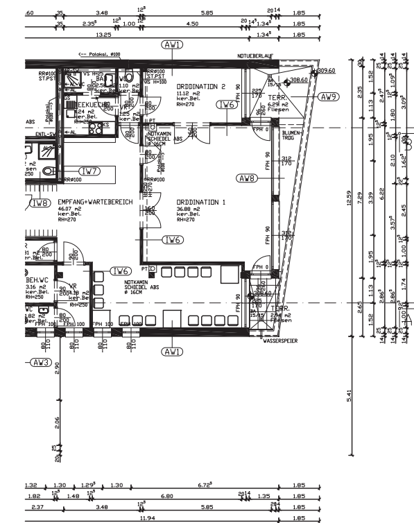
GRUNDRISS: OBERGESCHOSS
