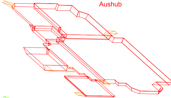
Schüttung
