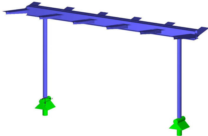
Vordach Vorkai
